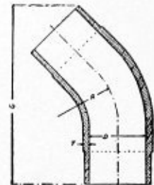
45° ELBOW
